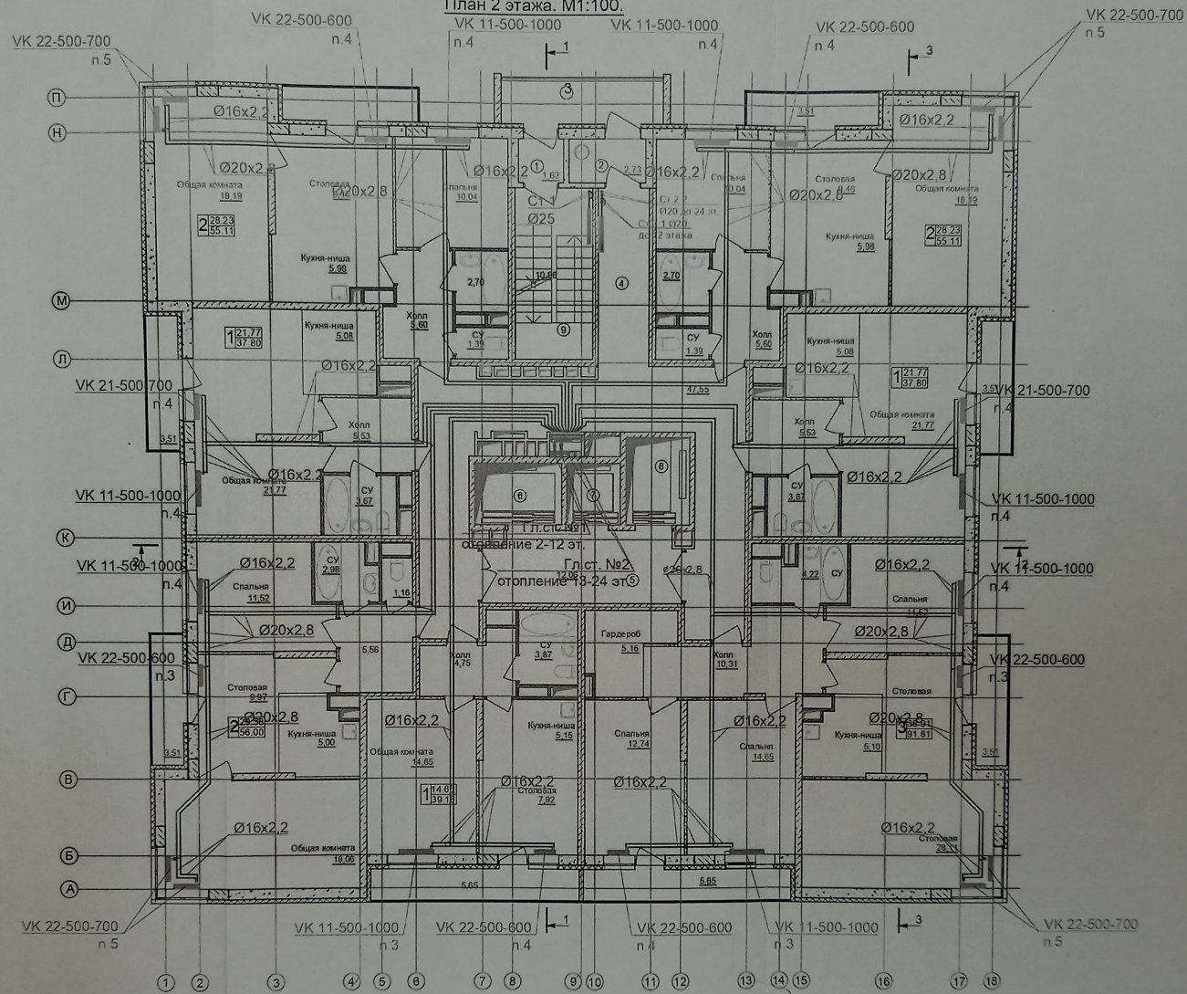
План 2 этажа. М1:100.
